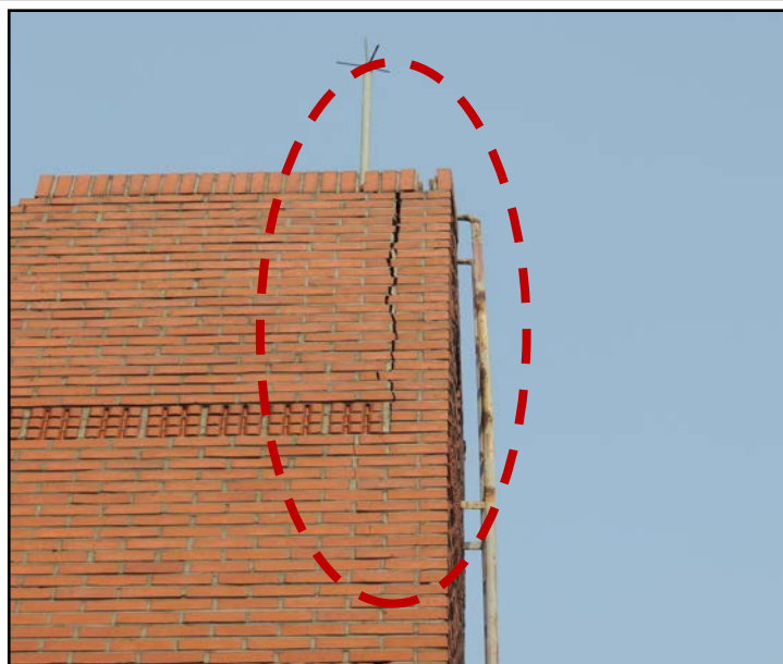
과천 향교말길 15-*번지 일반주택 외벽보수공사 (전)
