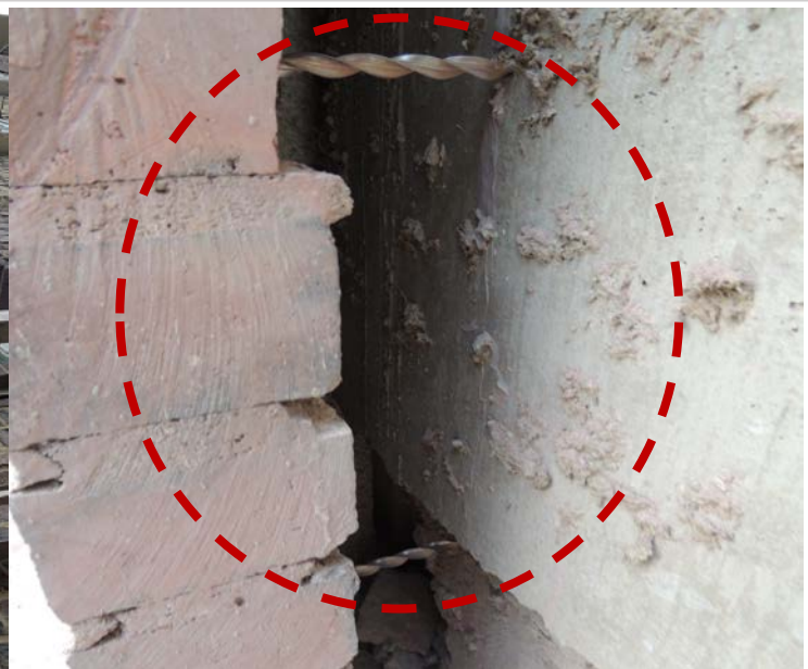
전북대학교 평화관 하이픽스 보강공사 (하이픽스 압입 후)
