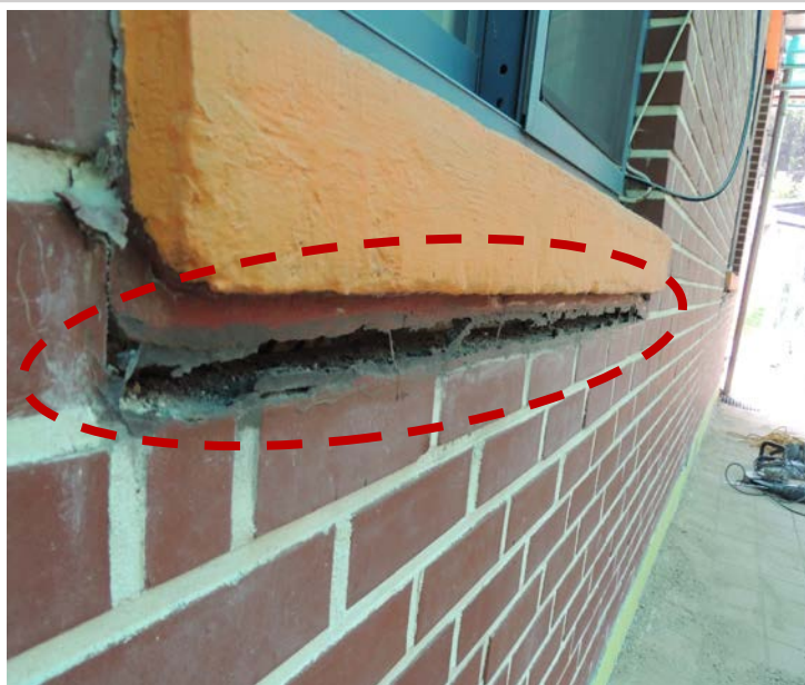
파주 삼성초등학교 외벽보수공사 (처짐 현상 시공전)
