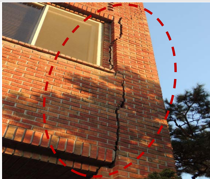
포항 한동대학교 현동홀 (지진붕괴)
