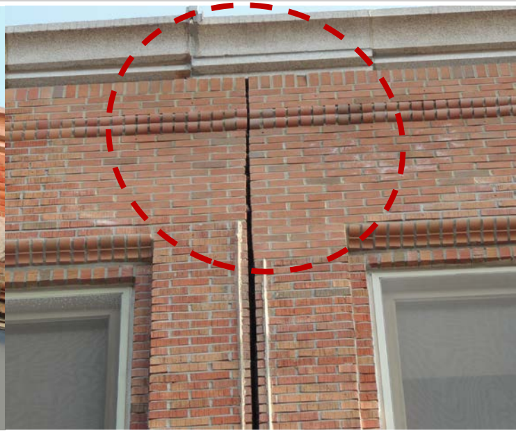
포항 한동대학교 현동홀 (후)
