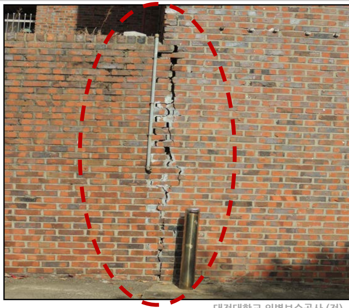
대전대학교 외벽보수공사 (전)
